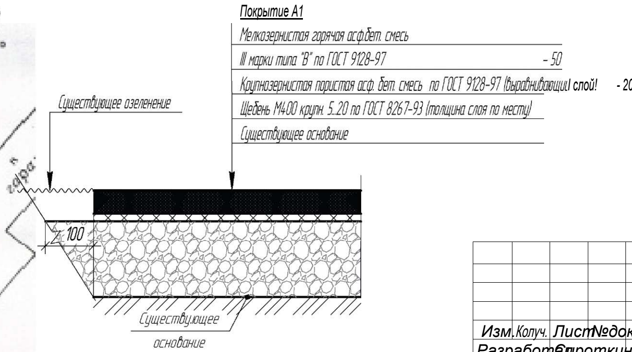
Узел устройства покрытия проездов, парковки и дорожек
